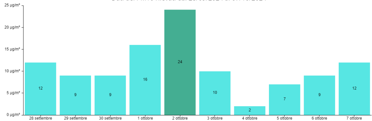
Dati del PM10 rilevati dal 28/09/2024 al 07/10/2024
