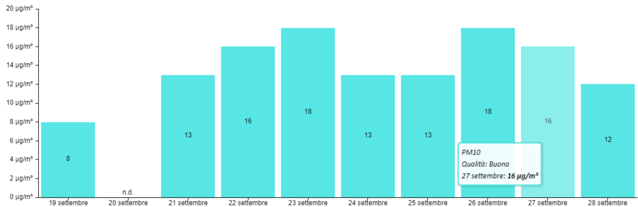
Dati del PM10 rilevati dal 19/09/2024 al 28/09/2024
