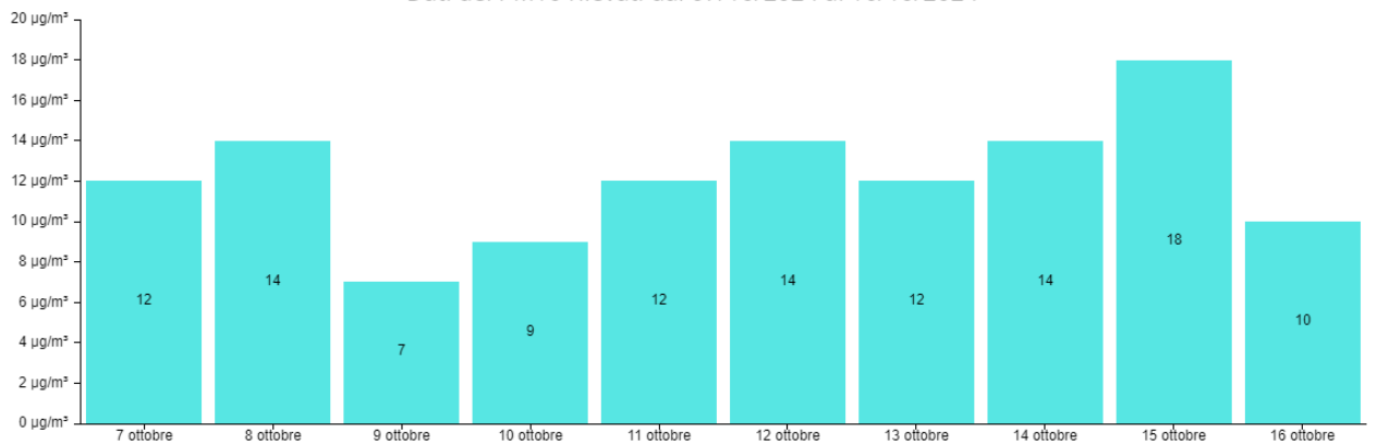
Dati del PM10 rilevati dal 07/10/2024 al 16/10/2024
