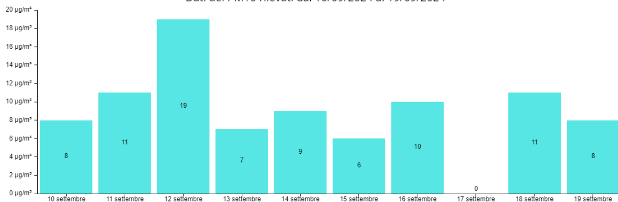
Dati del PM10 rilevati dal 10/09/2024 al 19/09/2024
