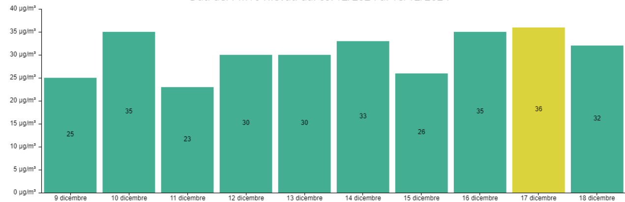
Dati del PM10 rilevati dal 09/12/2024 al 18/12/2024
