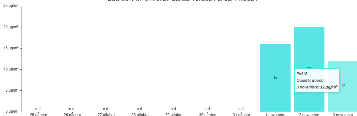
Dati del PM10 rilevati dal 25/10/2024 al 03/11/2024
