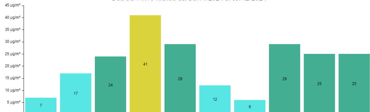
Dati del PM10 rilevati dal 30/11/2024 al 09/12/2024
