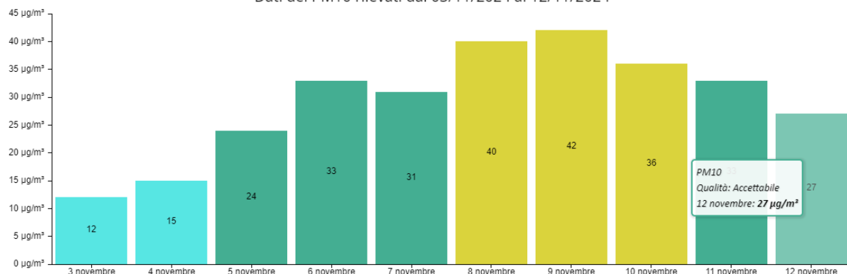
Dati del PM10 rilevati dal 03/11/2024 al 12/11/2024
