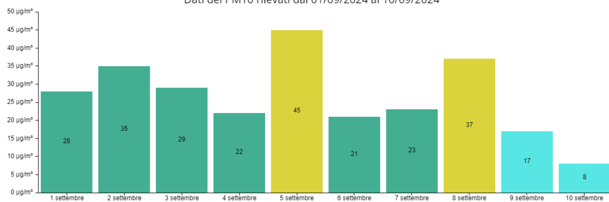
Dati del PM10 rilevati dal 01/09/2024 al 10/09/2024
