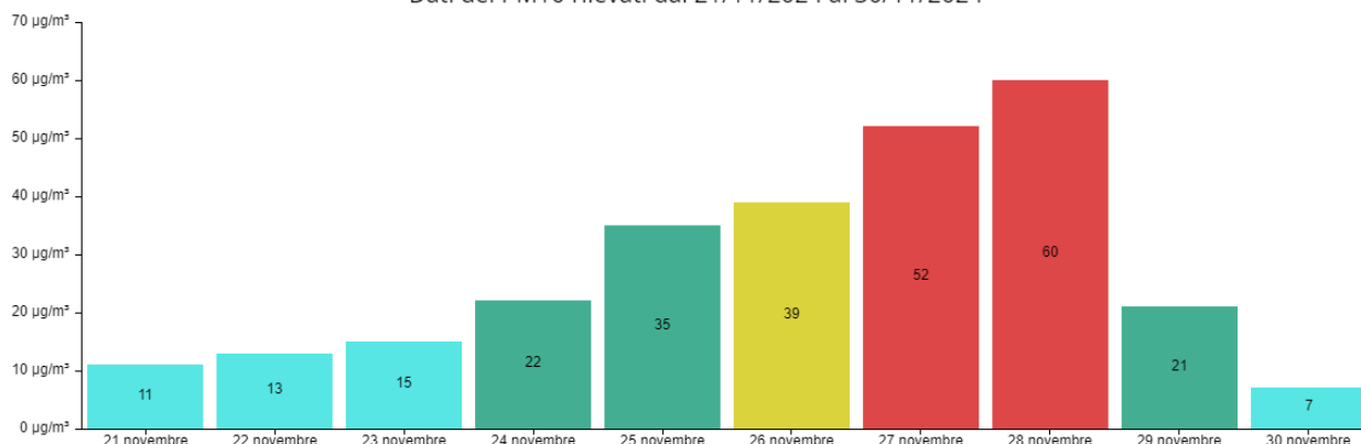
Dati del PM10 rilevati dal 21/11/2024 al 30/11/2024
