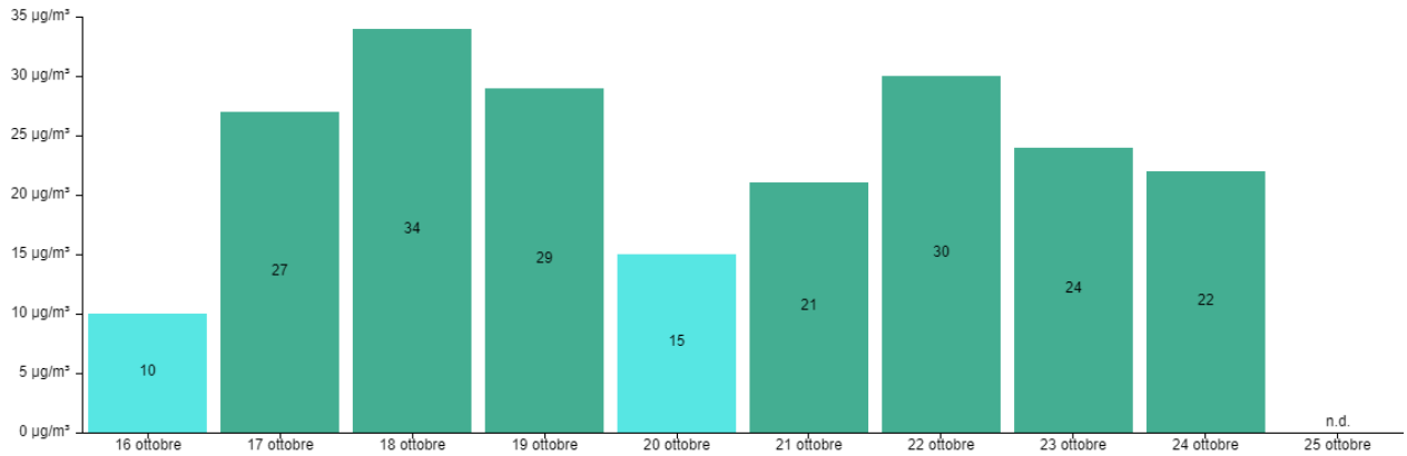
Dati del PM10 rilevati dal 16/10/2024 al 25/10/2024
