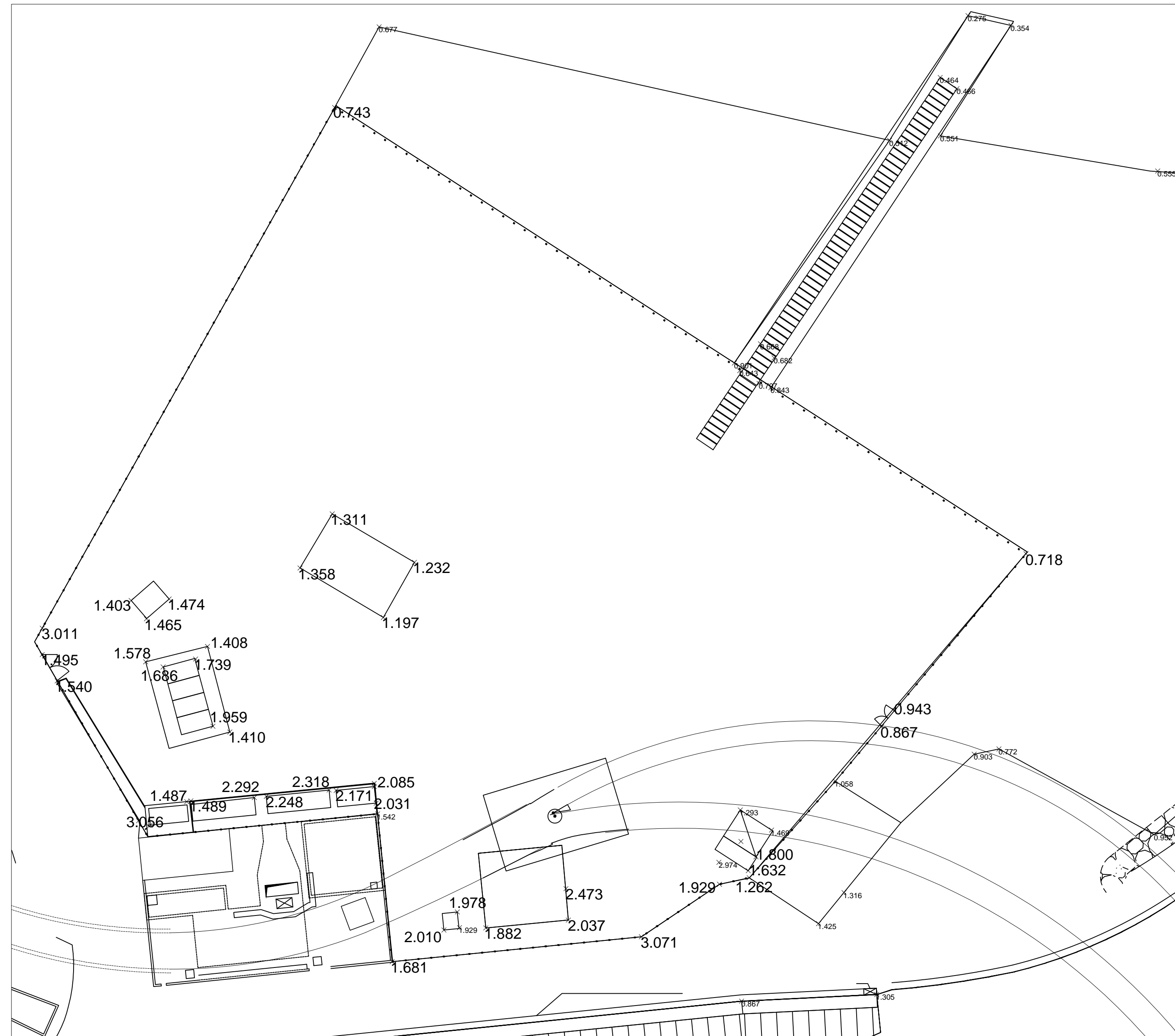
Rilievo planimetrico dello stato di fatto _ scala 1:500
