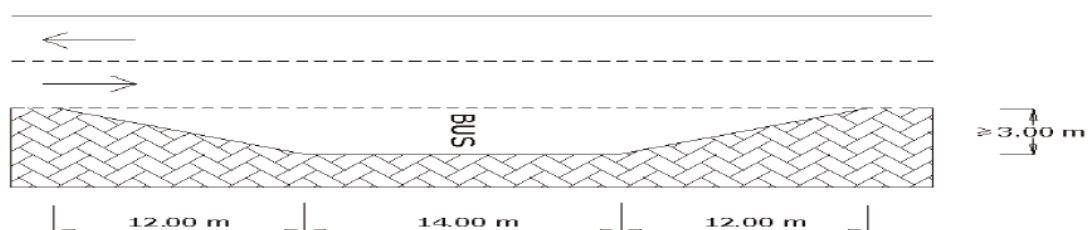
Figura 1 - Golfo di fermata esterno alla carreggiata
