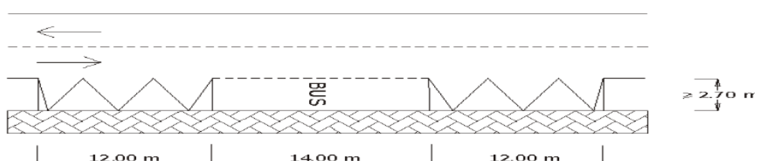
Figura 2 - Fermata in carreggiata
