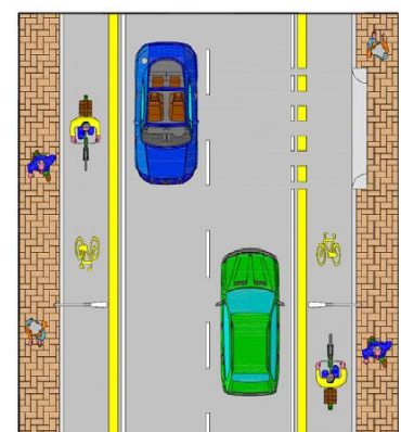
Figura 5 - esempio di pista ciclabile su corsia riservata
